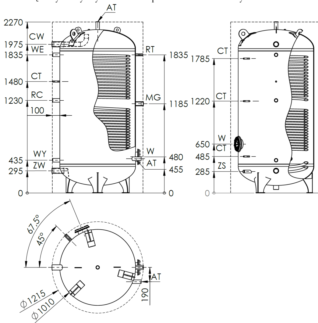
Rys.1 Budowa wymiennika WDP PC 1500
