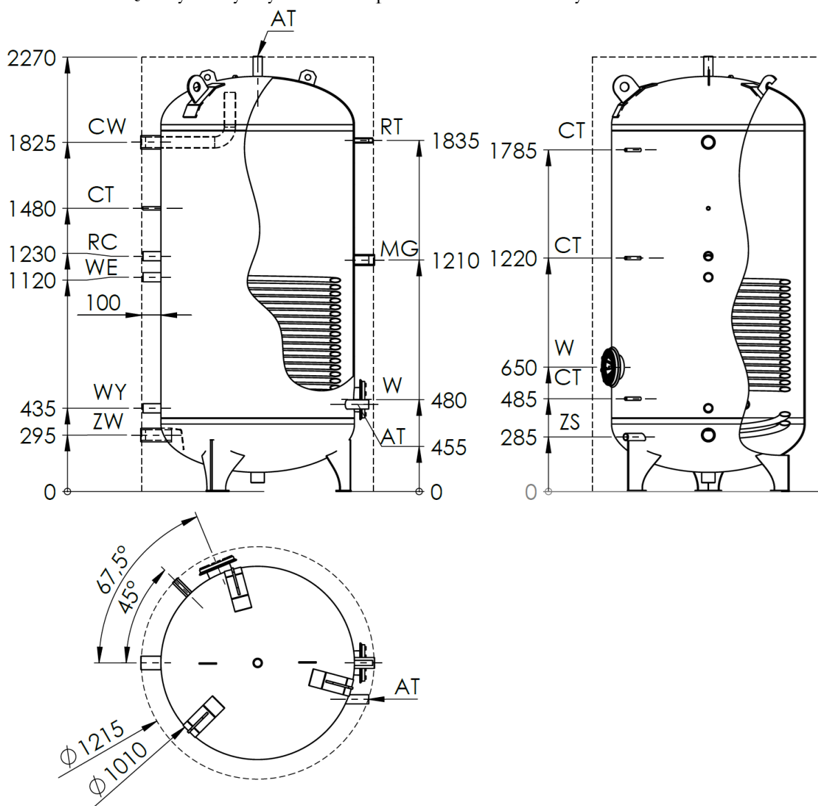
Rys.1 Budowa wymiennika WDP1 1500
