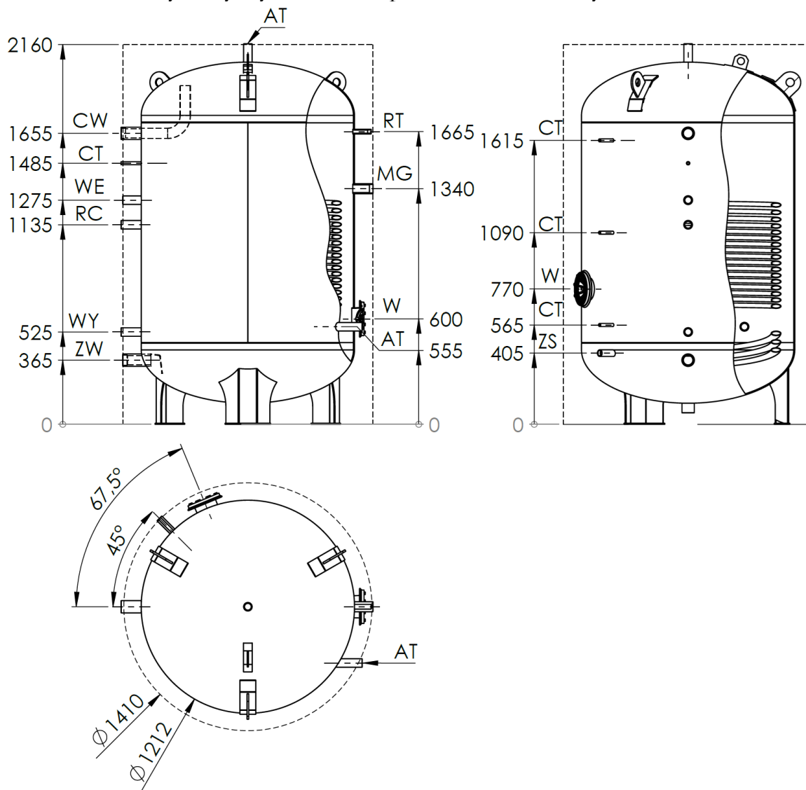
Rys.1 Budowa wymiennika WDP1 2000
