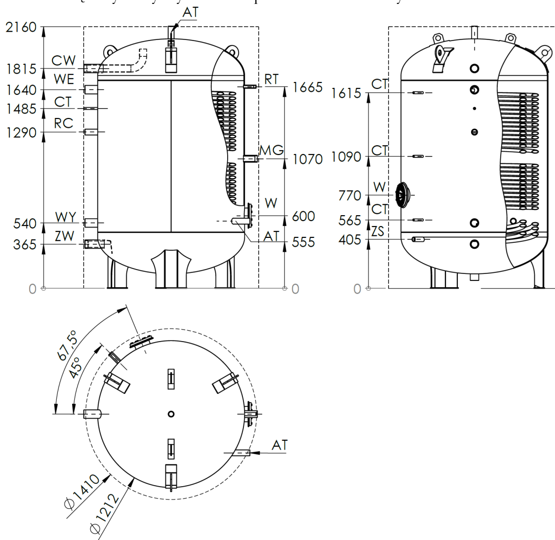
Rys.1 Budowa wymiennika WDP MEGA MAX 2000
