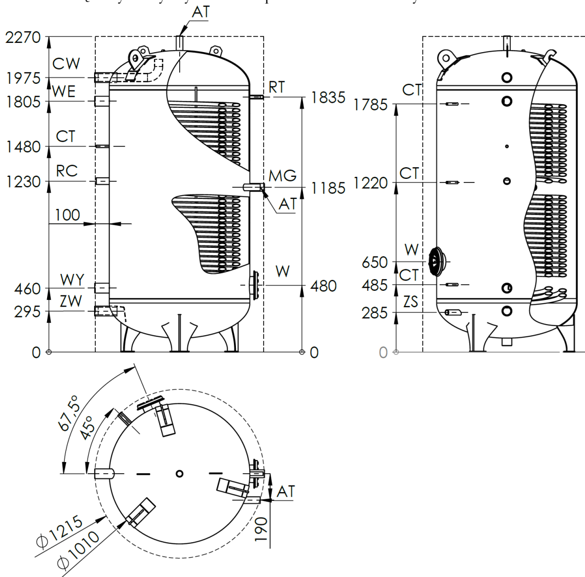
Rys.1 Budowa wymiennika WDP MEGA MAX 1500
