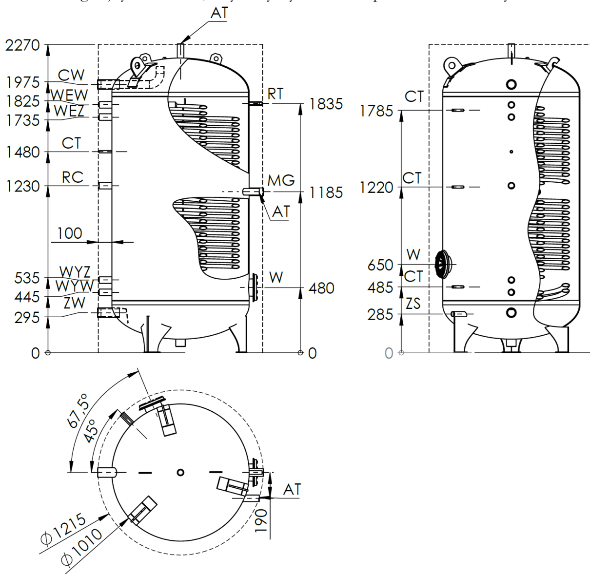
Rys.1 Budowa wymiennika WDP MAX DUO 1500
