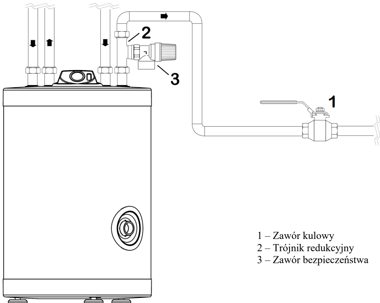
Rys. 3. Montaż zaworu bezpieczeństwa na trójniku redukcyjnym.
