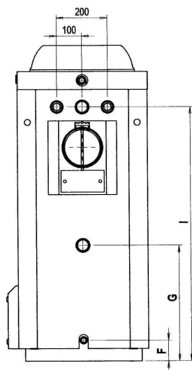
Rys.2 Wymiary kotłów EKO-KWR 15-30
