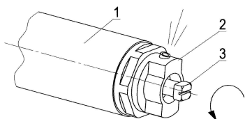
Rys.10 Odpowietrznik
