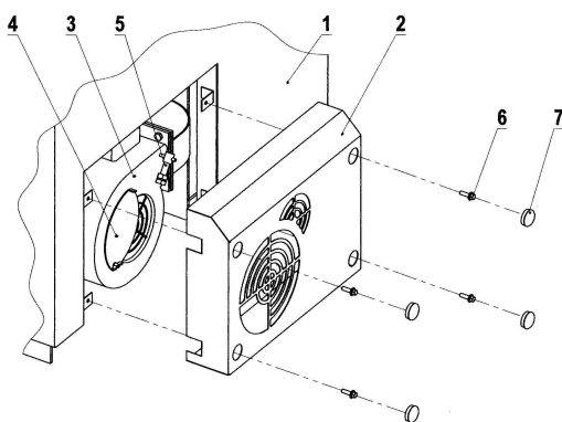
Rys.4 Wentylator nadmuchowy
