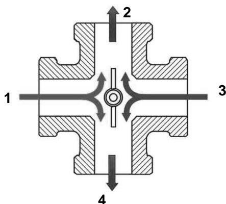
Rys.7. Czterodrogowy zawór mieszający
