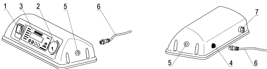
Rys. 3 Panel sterujący
