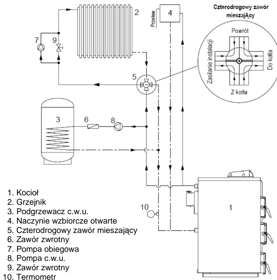
Rys.9. Przykładowy schemat podłączenia kotła do systemu grzewczego c.o. i c.w.u. z wykorzystaniem czterodrogowego zaworu mieszającego.
