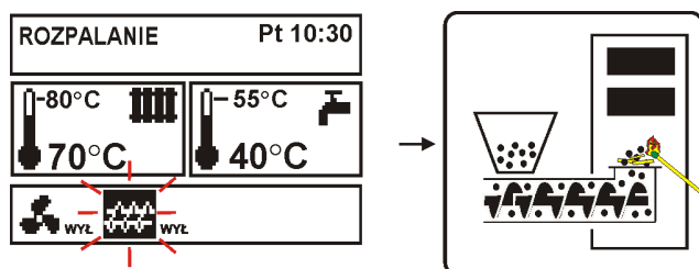
Rys. 7 Wyłączenie podajnika w rozpalaniu
