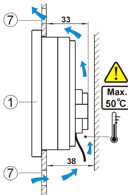
Rys. 29 Warunki zabudowy panelu, gdzie: 1 - panel, 7 - otwory wentylacyjne do cyrkulacji powietrza (uwaga: otwory nie mogą zmniejszać wymaganego stopnia ochrony IP; otwory wentylacyjne nie są wymagane jeśli graniczna temperatura otoczenia panelu nie jest przekroczona; otwory wentylacyjne nie zawsze mogą zagwarantować obniżenie temperatury otoczenia panelu w takim przypadku stosować inne metody),
