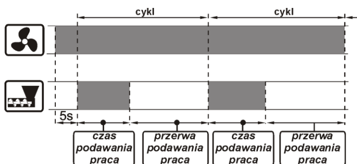
Rys. 11 Cykle pracy nadmuchu i podajnika w trybie PRACA
