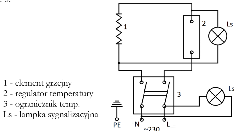
Rys. 3. Schematy elektryczne ogrzewaczy.
